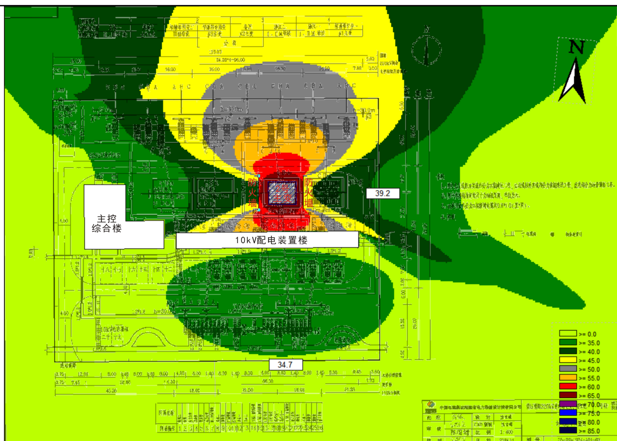
图 4-3 渭阳 220kV 变电站 2 号主变建成投运后噪声贡献等声级线图（围墙上方 0.5m）
