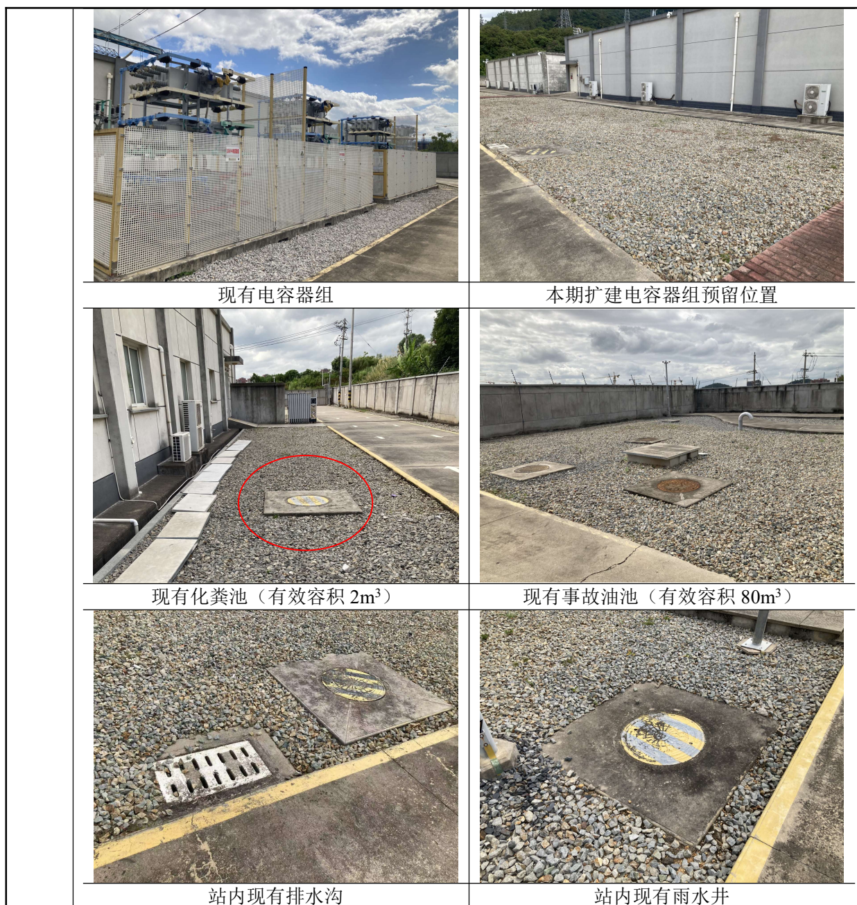
图 2-1 渭阳 220kV 变电站站内现状照片
