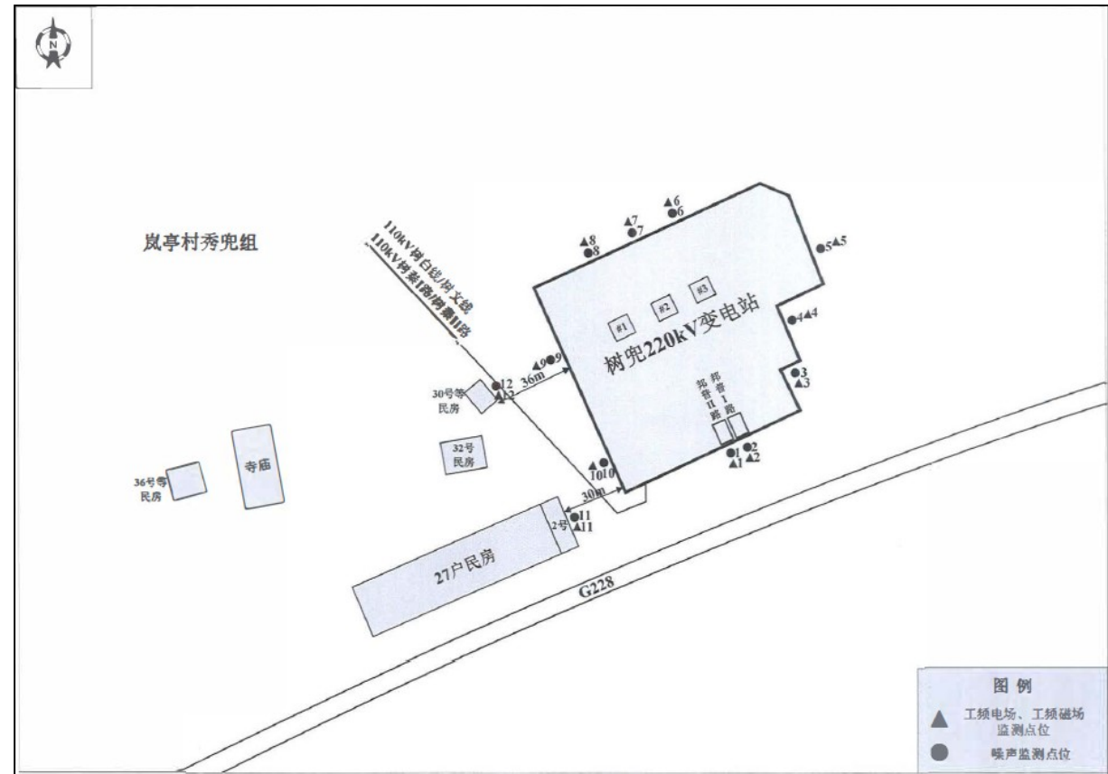
图 A-2 树兜 220kV 变电站监测布点示意图
