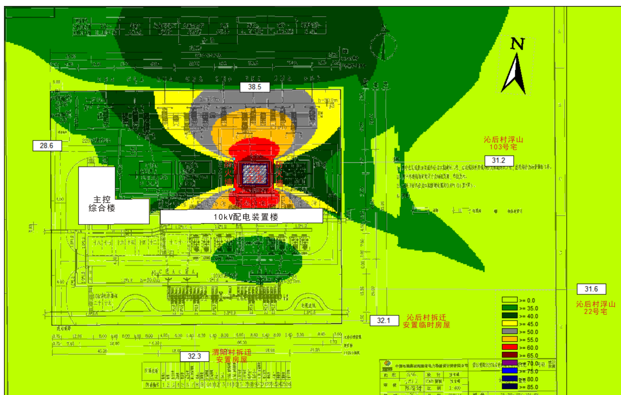
图 4-4 渭阳 220kV 变电站 2 号主变建成投运后噪声贡献等声级线图（地面 1.2m）
